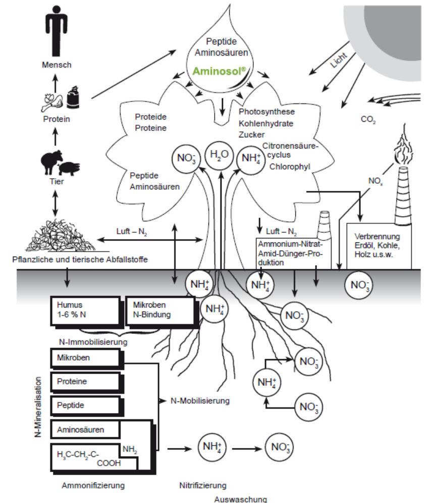
Der oberirdische und der unterirdische Stickstoff-Kreislauf
